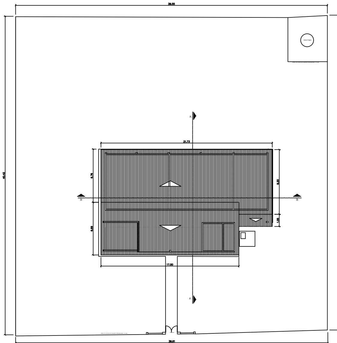
PLANTA DE COBERTURA - EMEF. JOSÉ ÍRIS COTIAS DE OLIVEIRA ESCALA 1/100
