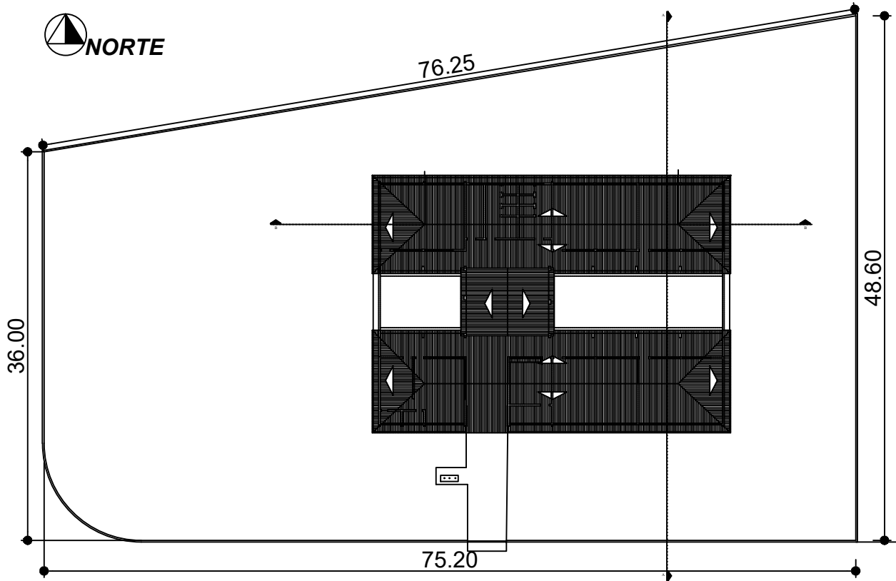
PLANTA DE COBERTURA - EMEF. PROFESSOR E JORNALISTA LUIZ ANTÔNIO BARRETO ESCALA 1/75
