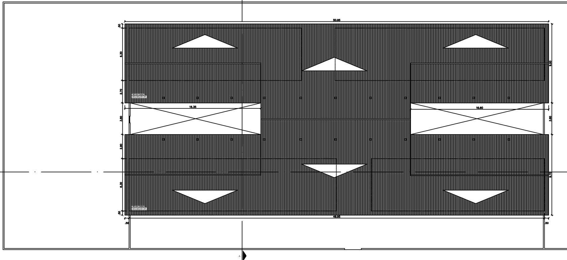
PLANTA DE COBERTURA ESCALA 1/100
